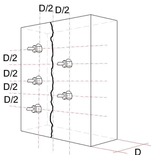
DETALHE DE INSTALAÇÃO DOS BICOS DE INJEÇÃO
