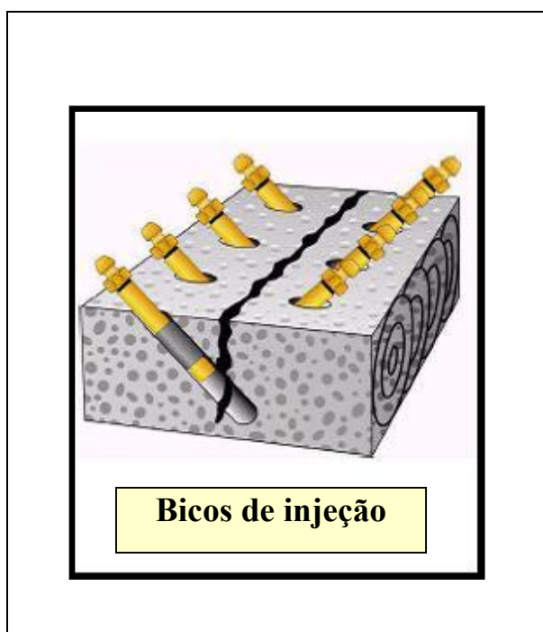
DETALHE DE INSTALAÇÃO DOS BICOS DE INJEÇÃO
