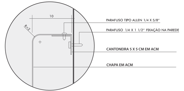
DETALHE 05
