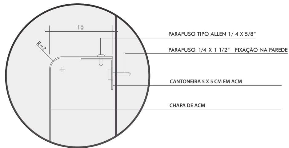
DETALHE 01
