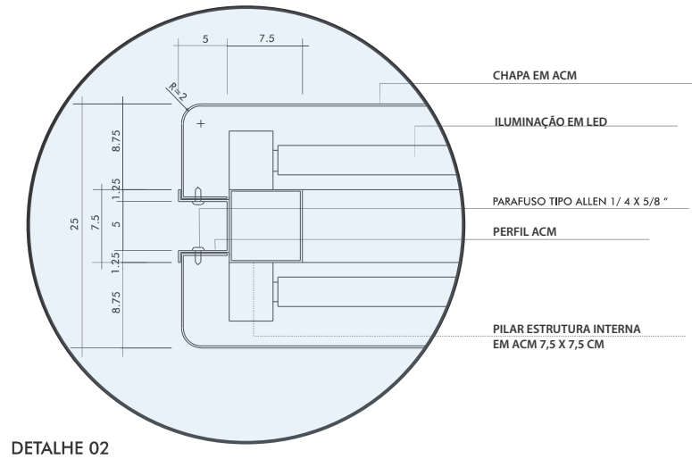
DETALHE 02
