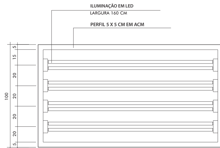
VISTA INTERNA
