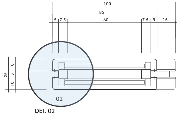
PLANTA NÍVEL MÉDIO
