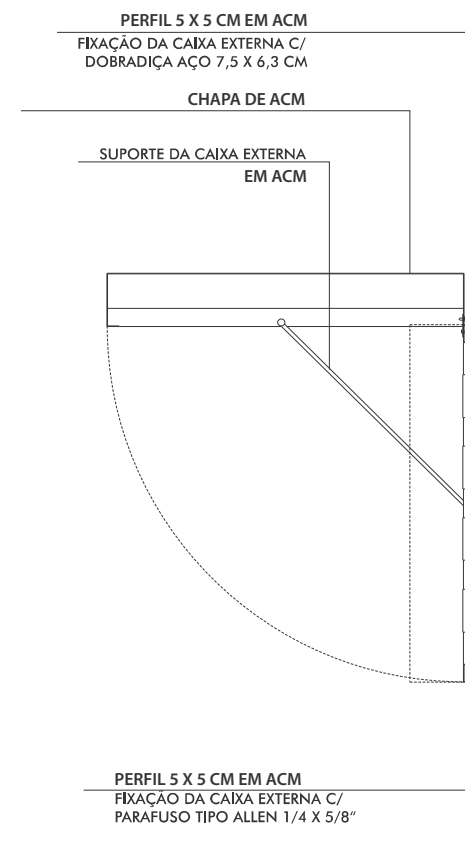
CORTE
