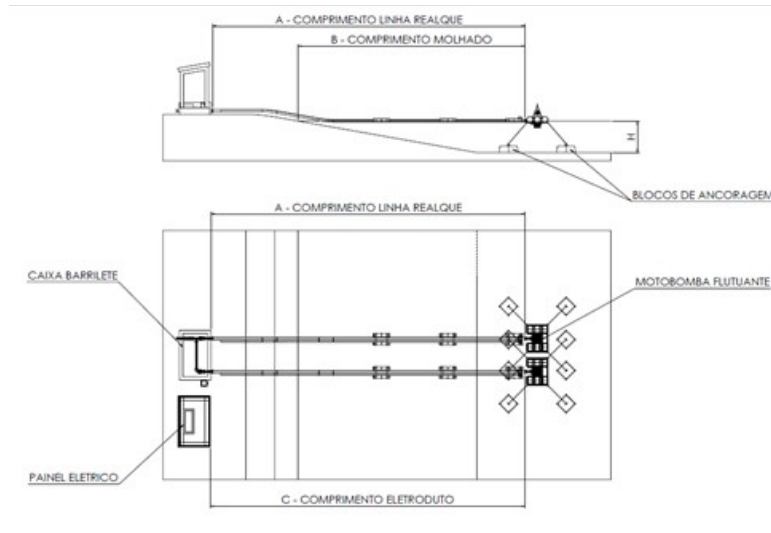
Figura 02- Dimensões gerais
